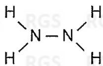
\text{N}_2\text{H}_4
