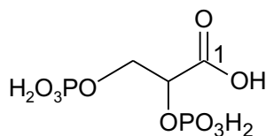
2,3-DPG
